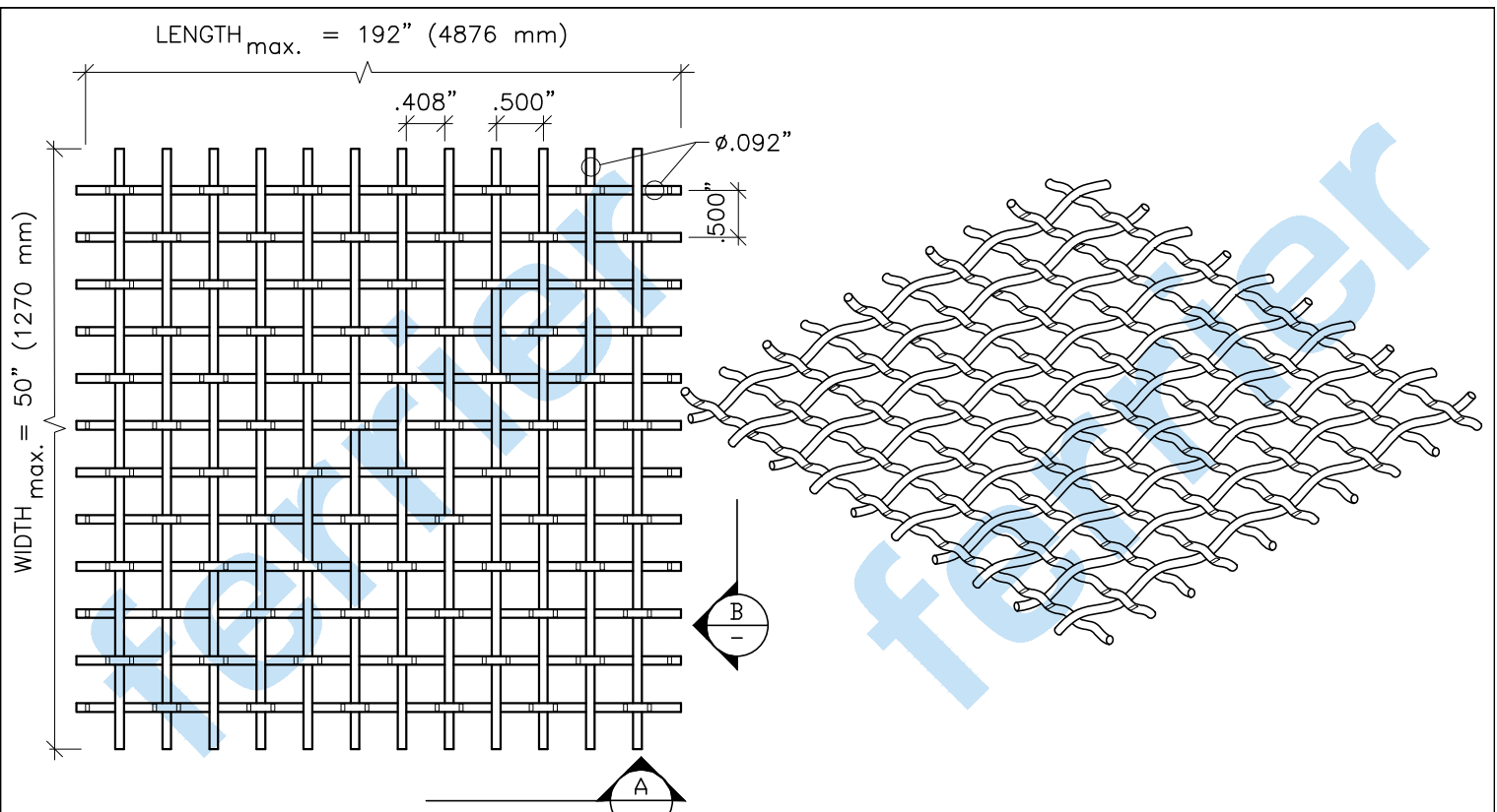
PLAN SCALE: 6"=1'-0"
