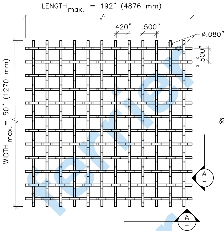
PLAN SCALE: 6"=1'-0"
