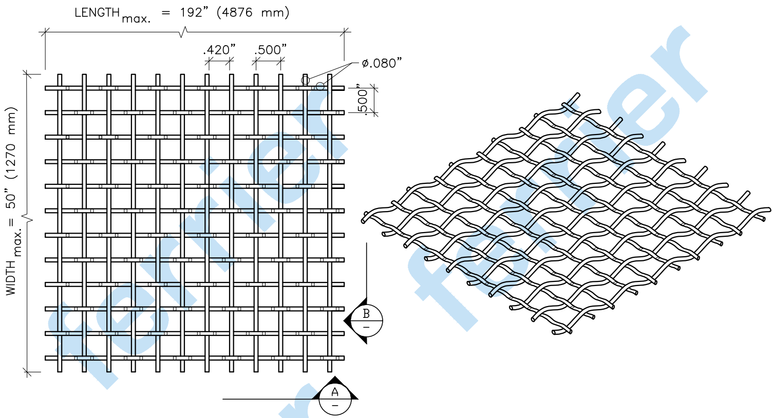
PLAN SCALE: 6"=1'-0"
