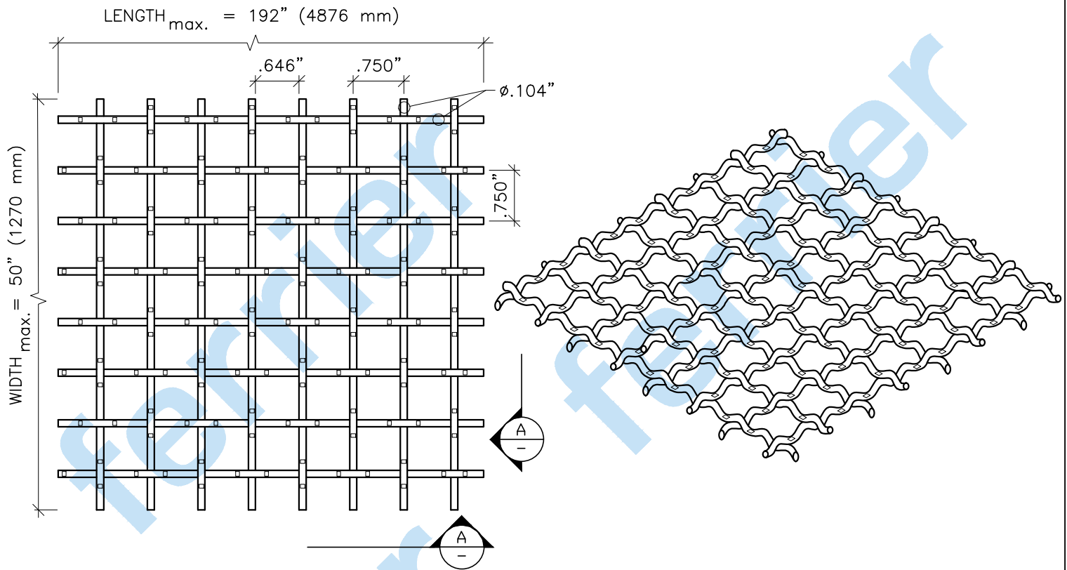
PLAN SCALE: 6"=1'-0"
