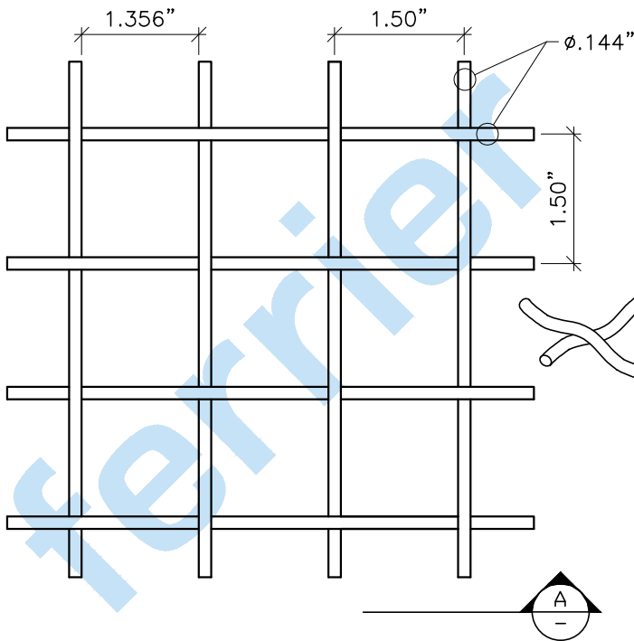
PLAN SCALE: 6"=1'-0"
